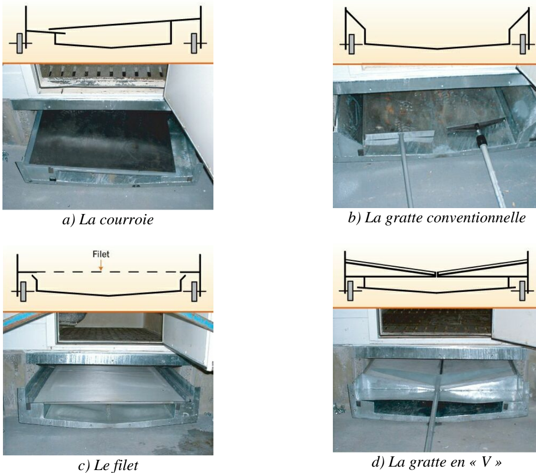
Figure 9 : Les systèmes expérimentaux de séparation sous les lattes
