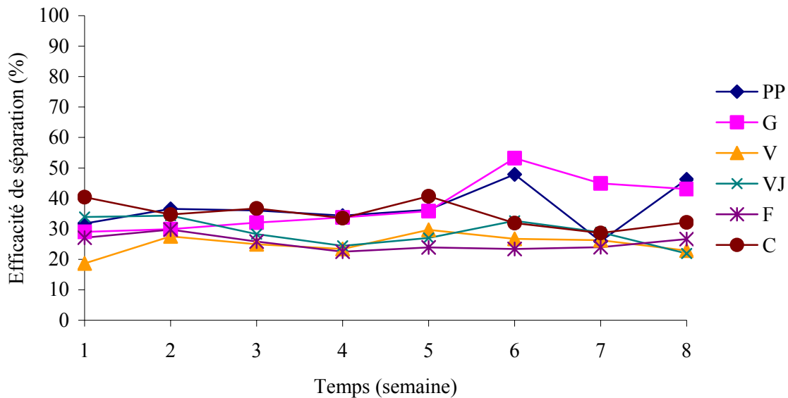
Figure 18 : Évolution de l'efficacité de séparation de l'azote ammoniacal en fonction des différents traitements
