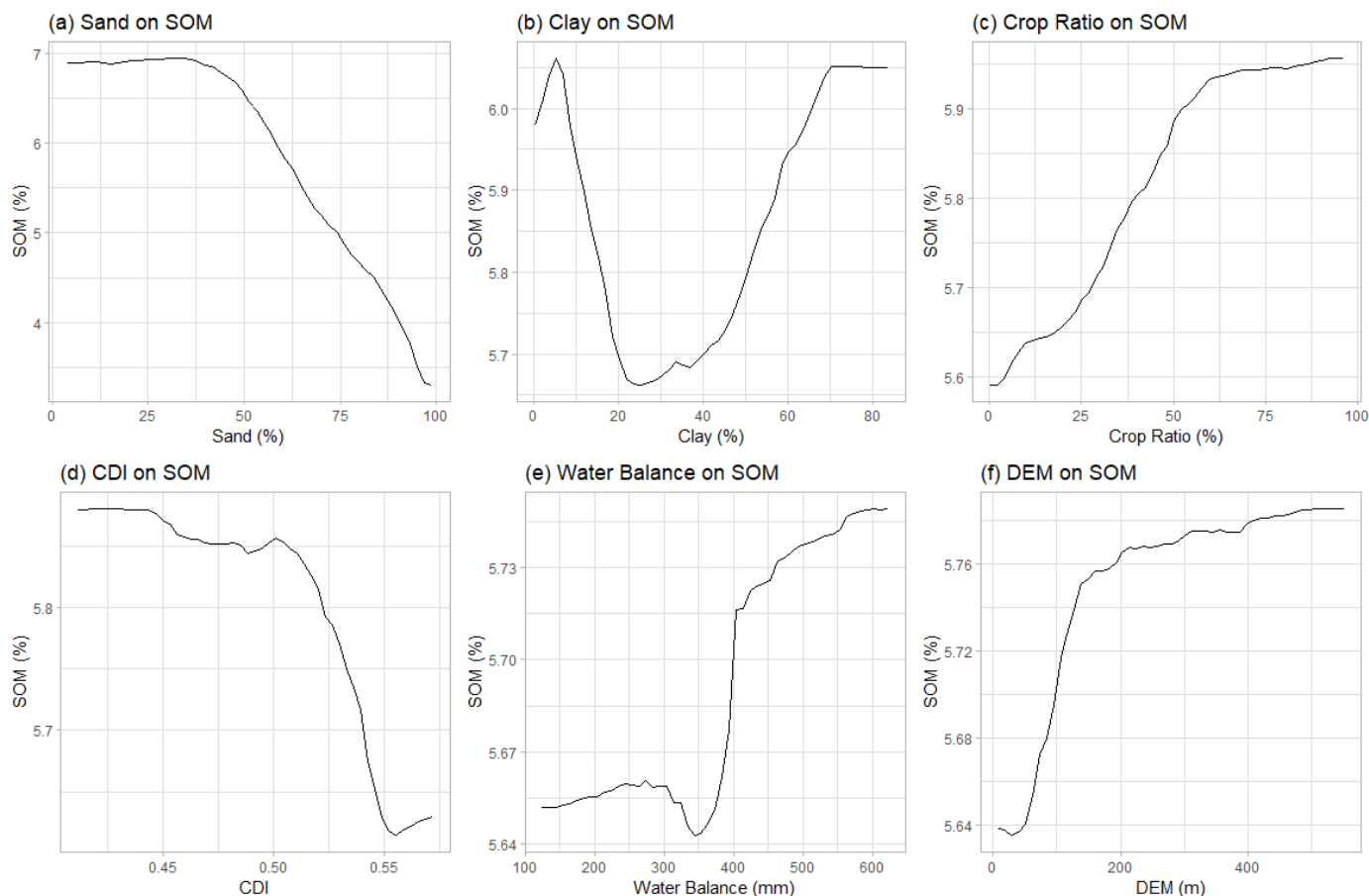
Figure 23 : Graphiques des dépendances partielles ( partial dependence plot ) entre la teneur en MOS et les variables prédictives les plus importantes, soit la teneur en sable (a), la teneur en argile (b), le ratio de cultures pérennes (c), le CDI (d), le bilan hydrique (e) et le modèle numérique de terrain (DEM) (f).
