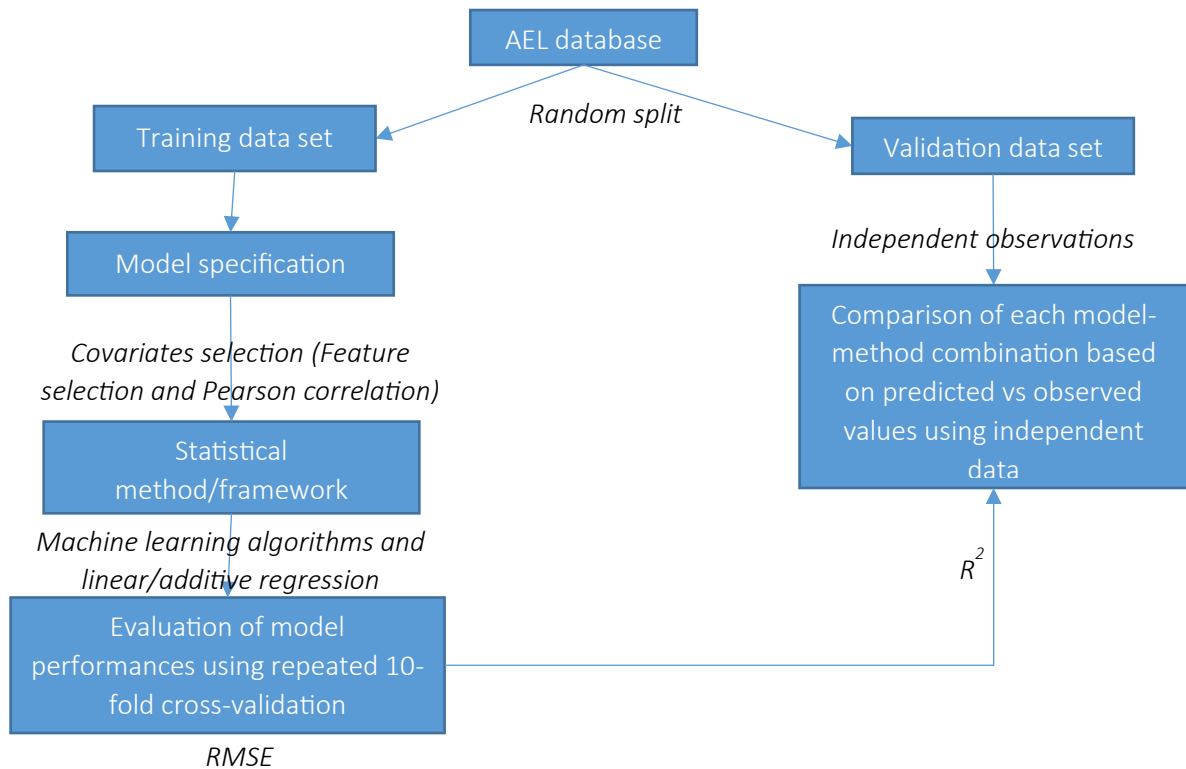
Figure 19 : Schéma des principales étapes du processus de modélisation utilisé.
