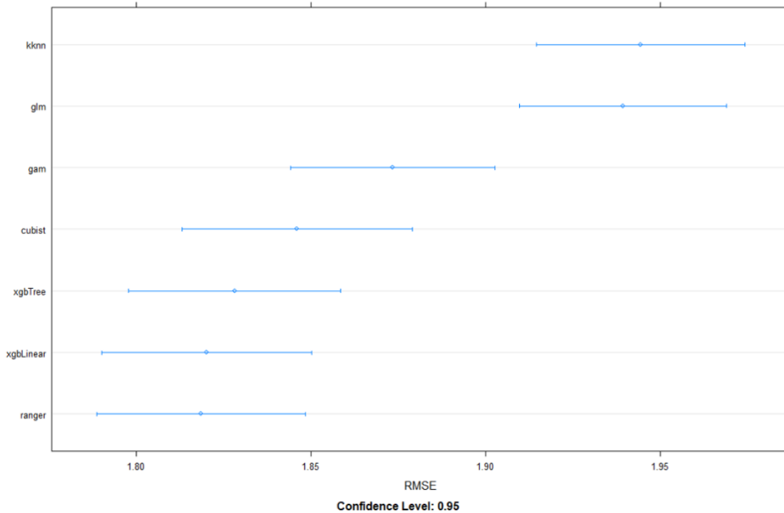
Figure 20 : Erreur quadratique moyenne (RMSE, %) et son intervalle de confiance à 95 % pour la prédiction de la matière organique du sol (MOS). Acronymes des méthodes statistiques : KKNN = k le plus proche voisin (méthode pondérée) ; GLM = modèle linéaire généralisé ; GAM = modèle additif généralisé ; Cubist = Algorithme cubiste ; XGBtree = Extreme gradient boosting trees ; XGBlinear = Extreme gradient boosting linear ; Ranger = forêts aléatoires.
