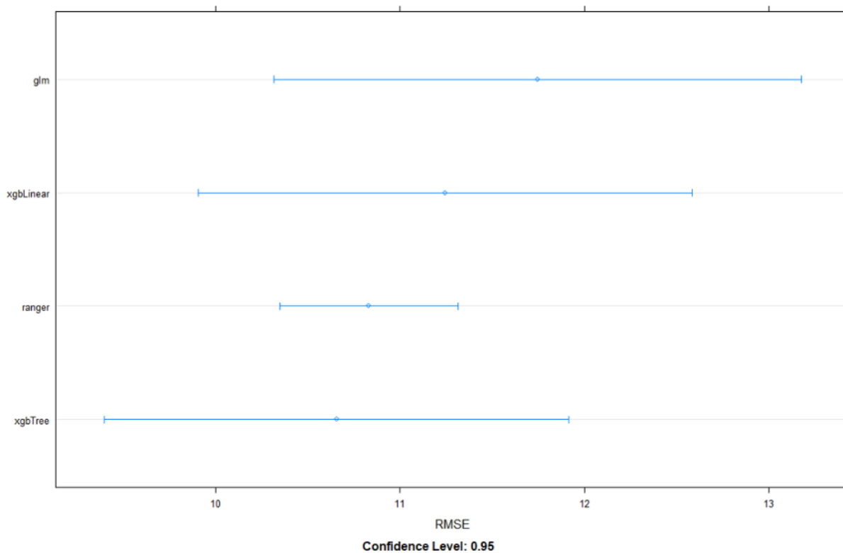
Figure 24 : Erreur quadratique moyenne (RMSE en %) et son intervalle de confiance à 95 % de la prédiction du ratio de cultures pérennes.
